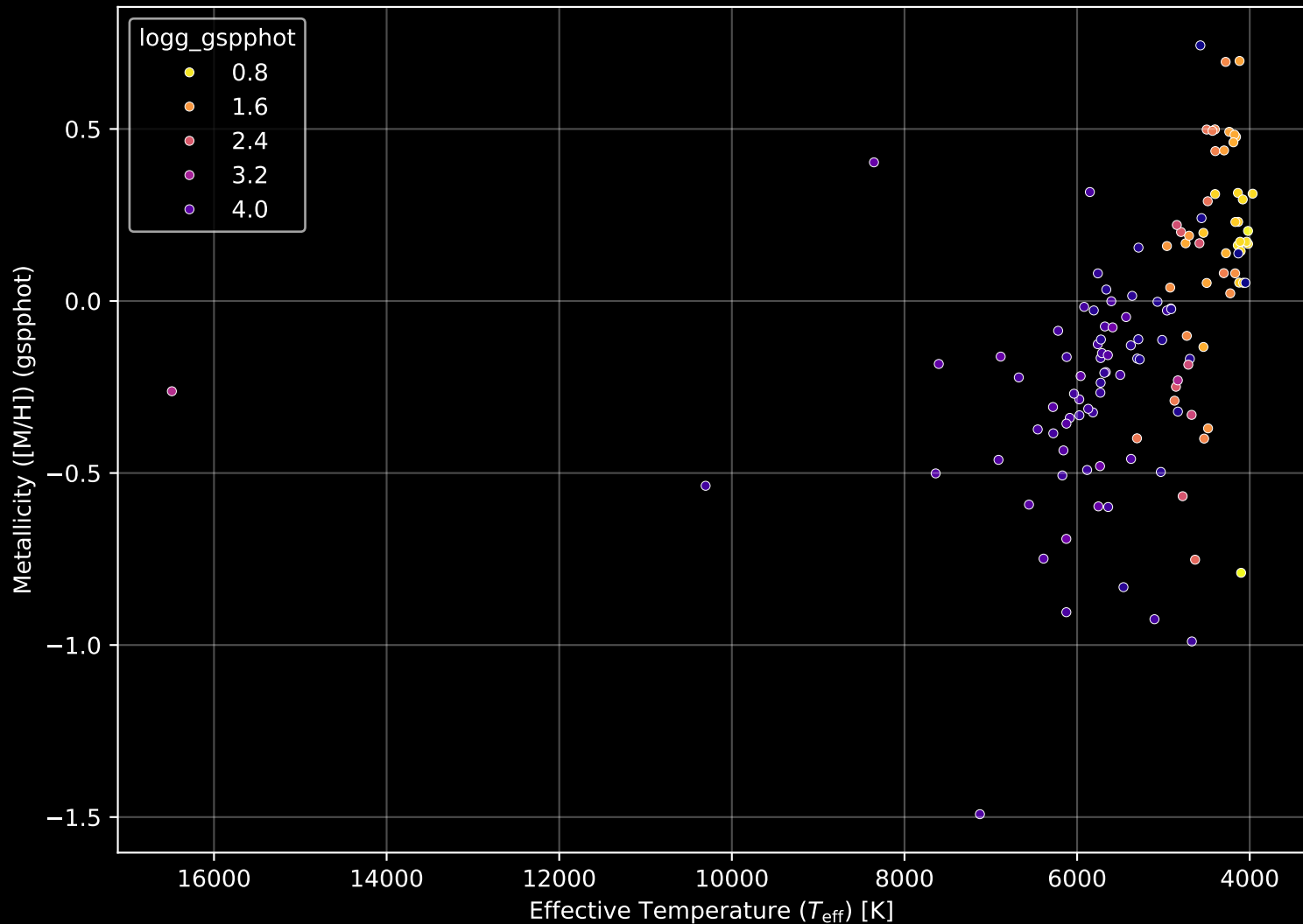
APOGEE DR17 Field: [277-33-O_TESS] Stellar Population Parameters (n= 126)
